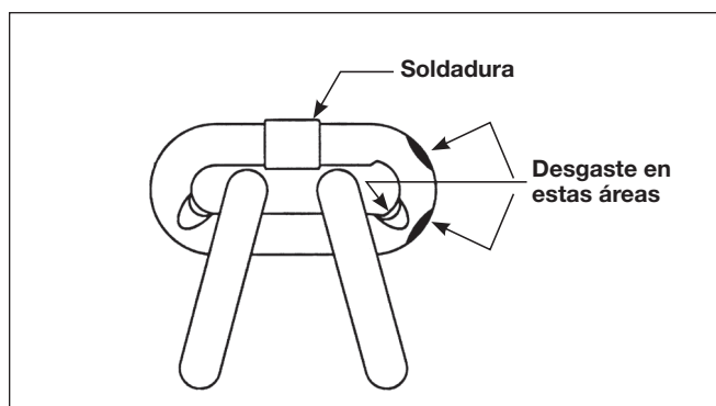
Figura 6 - Inspección de la cadena
