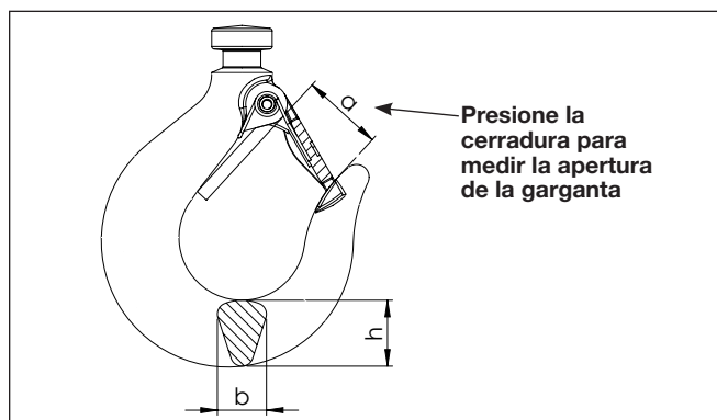
Figura 5 - Inspección del gancho
